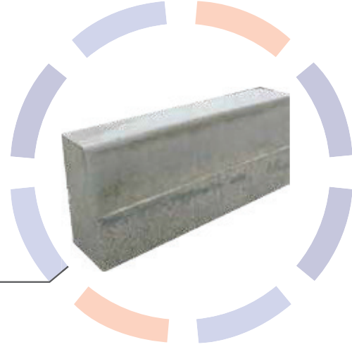
Belediye Tipi Bordür 150x300x700 mm 1 Ad. = 65 Kg.
