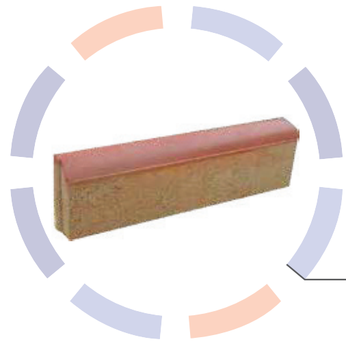
Geçmeli Yarım Oval Bahçe Bordürü Kırmızı 120x200x700 mm 1 Ad. = 40 Kg.
